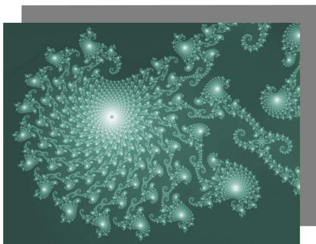
FRATTALE DI MANDELBROT
